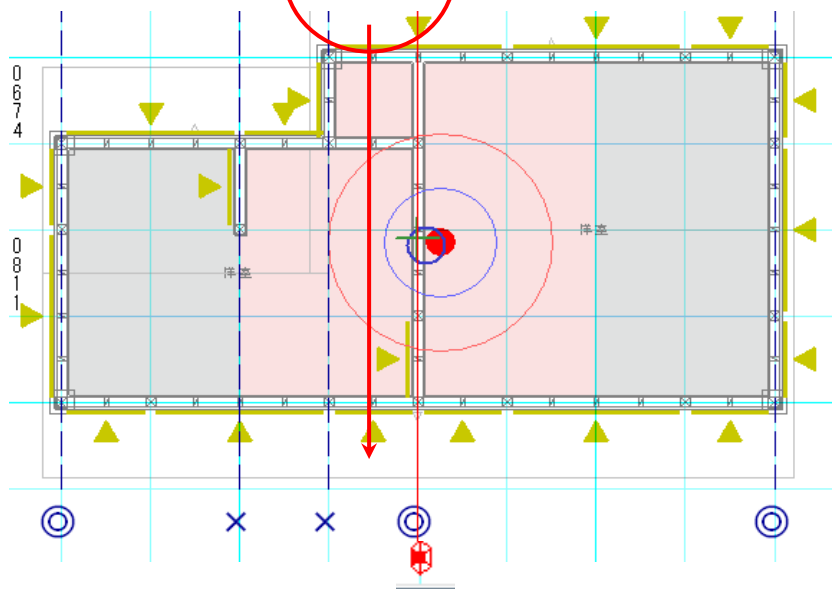
壁線候補追加後
