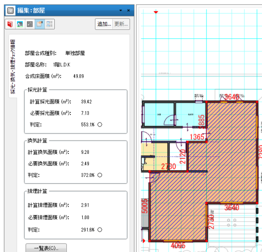
居室を選択した状態
