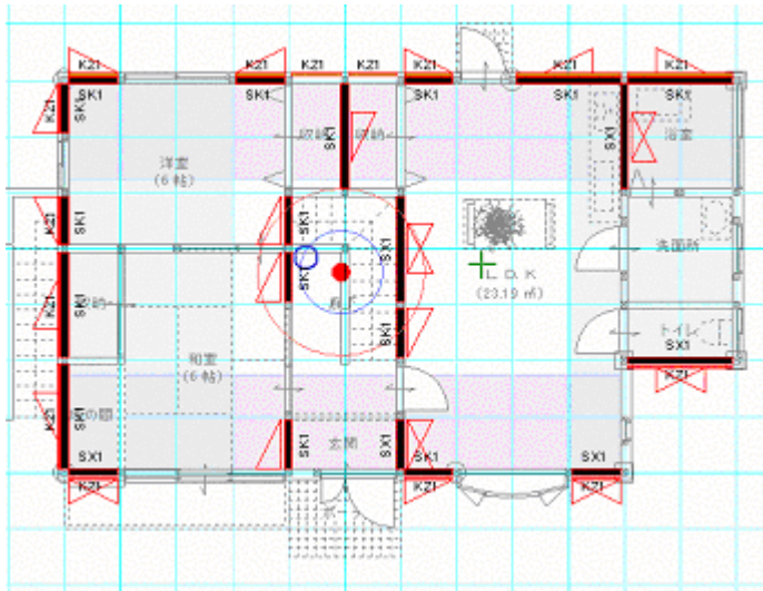
一部を矢形に変更し、0.15 推奨円の範囲に入るように調整した例
